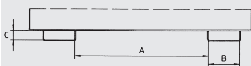
Dimensions intérieures des fourreaux en mm
