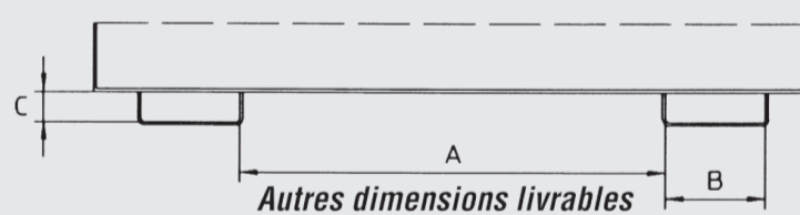
Dimensions intérieures des fourreaux en mm
